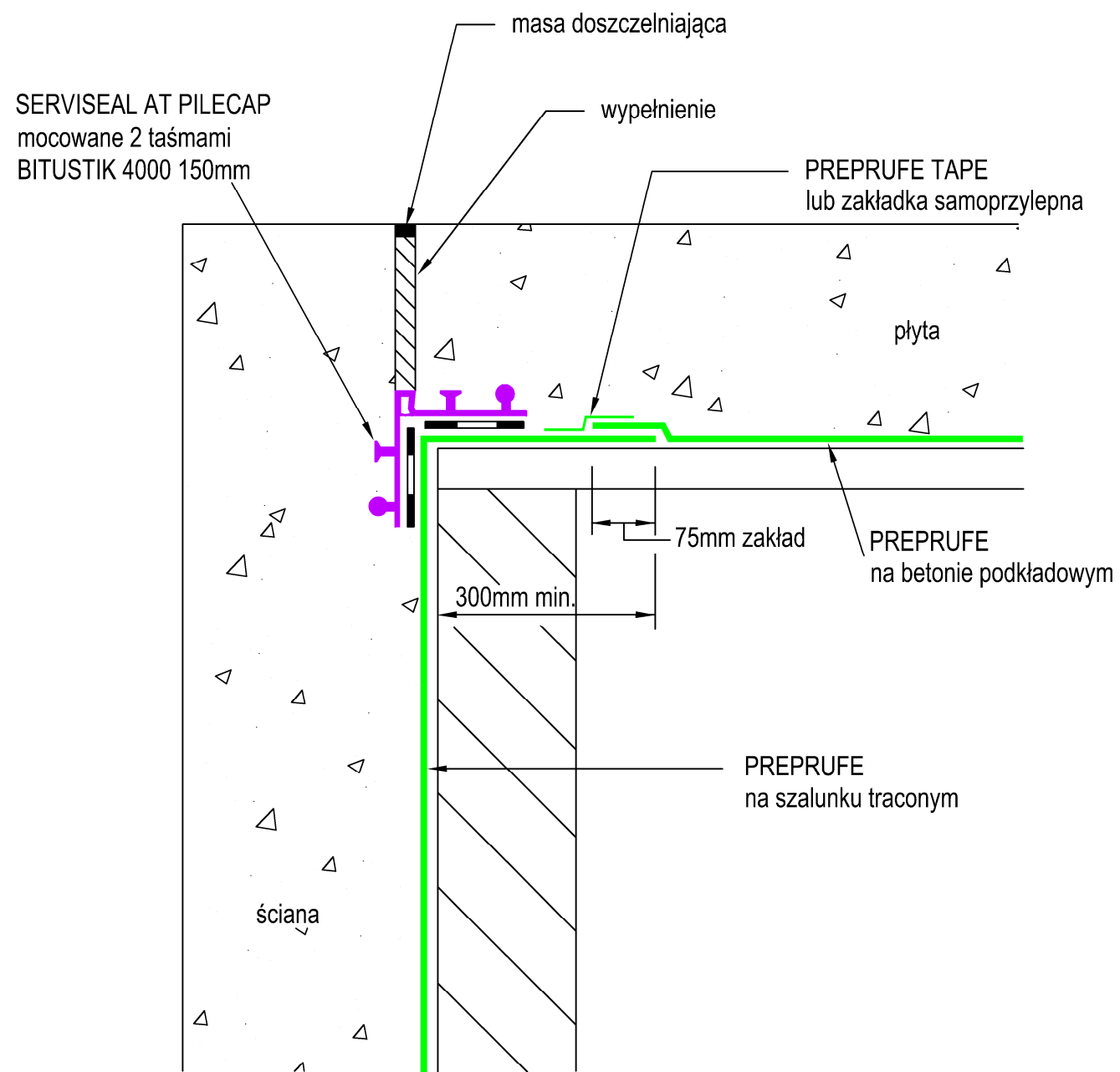
DETAL DYLATOWANEGO POŁĄCZENIA ŚCIANY Z PŁYTA PRZEKRÓJ
